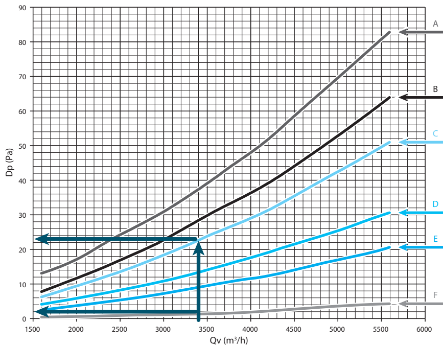
Graphique "Pertes de charge" Maestro MTL 64
