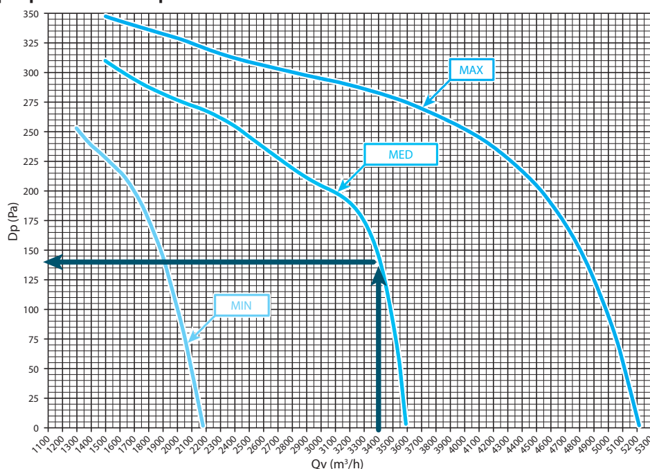
Graphique "Pression disponible" Maestro MTL 64
