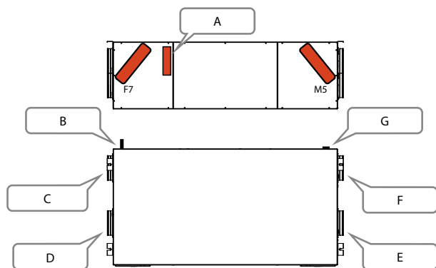
Configuration côté droit par défaut (vue de dessus)
