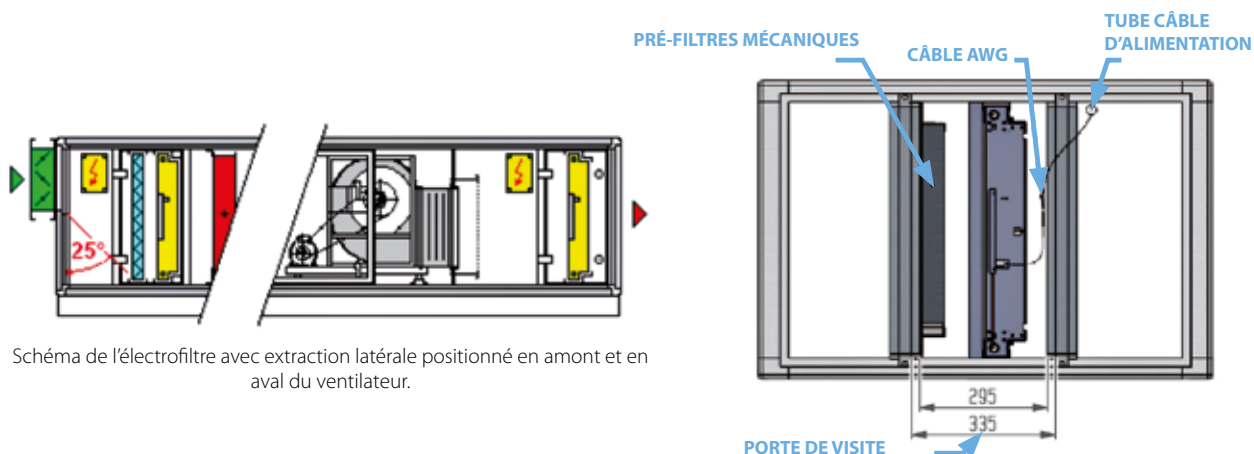
Encombrements de l'électrofiltre avec pré-filtre mécanique à extraction latérale.
