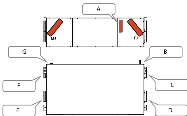
Configuration côté gauche en option (vue de dessus)
