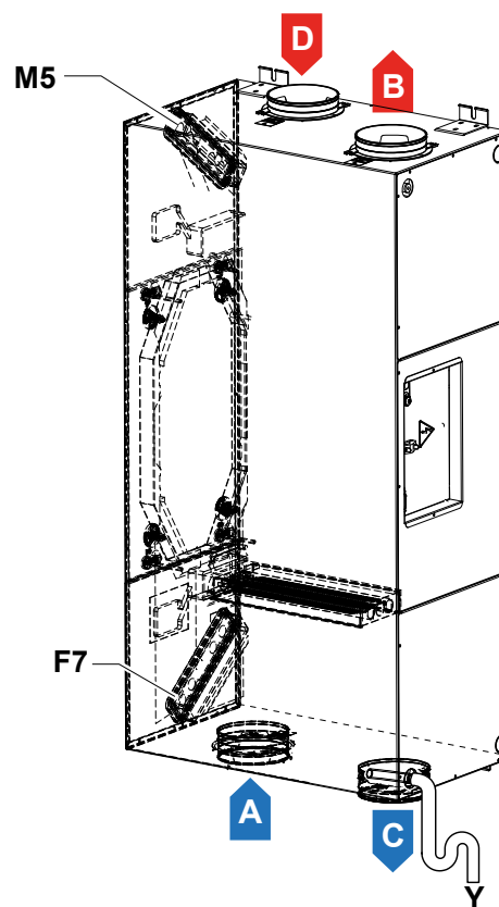
Configuration inversée finale
