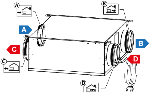
Unité horizontale ENY VAV (droite)
