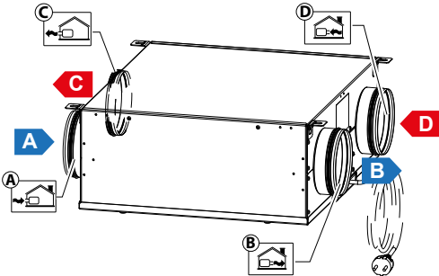
Unité horizontale ENY VAV (gauche)
