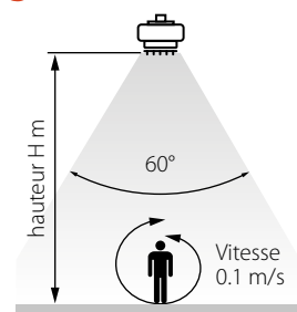
PORTÉE à 30° de chaque cote
