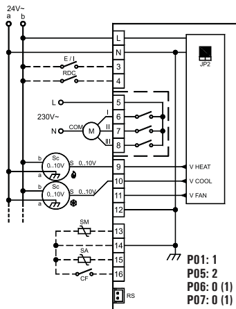
Fig. 10: Esquema de conexión para pilotaje de dos actuadores 0..10V à 24V ~ pour installation à 4 tubes et pilotage d'un moteur à trois vitesses à 230V.
