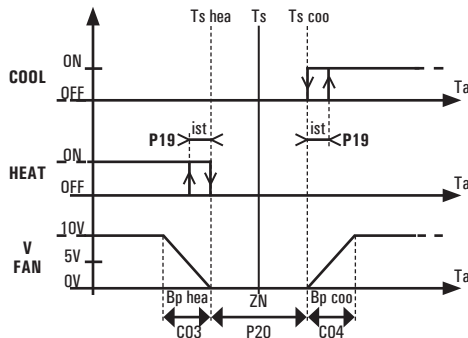
Fig. 15: Le schéma montre le pilotage des vannes dans un système à 4 tuyaux avec zone neutre. De façon analogue, la sortie de la vanne chaude ( HEAT ) d'un système à 2 tuyaux sera pilotée de la même manière ; dans ce cas-là, la T_s (température du point de consigne) coïncidera avec la T_s hea en hiver et avec la T_s coo en été. Le schéma ne tient pas compte de l'action éventuelle du temps d'intégration et présume que la sortie proportionnelle du ventilateur ( V FAN ) est configurée pour action directe ( P05=0 ) et pour un signal 0-10 V ( C15=0 ; C16=100 ). La sortie proportionnelle du ventilateur est toujours éteinte (0 V) quand la sortie de la vanne ( COOL ou HEAT ) est éteinte (ce cas n'est pas visible sur le schéma).
