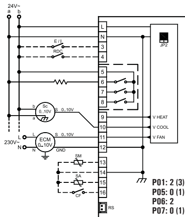
Fig. 11: Esquema de conexión para pilotaje de dos actuadores 0..10V à 24V ~ pour installation avec résistance d'intégration et pilotage proportionnel du ventilateur.
